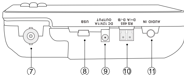
左侧接口图
